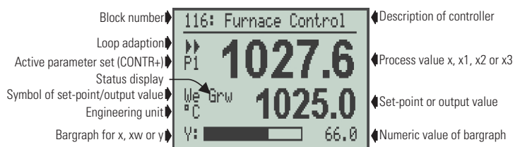
Fig. 2 Operating display for a controller (CONTR, CONTR+)
